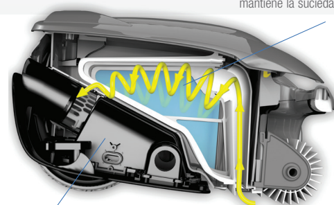
Motor inclinado
